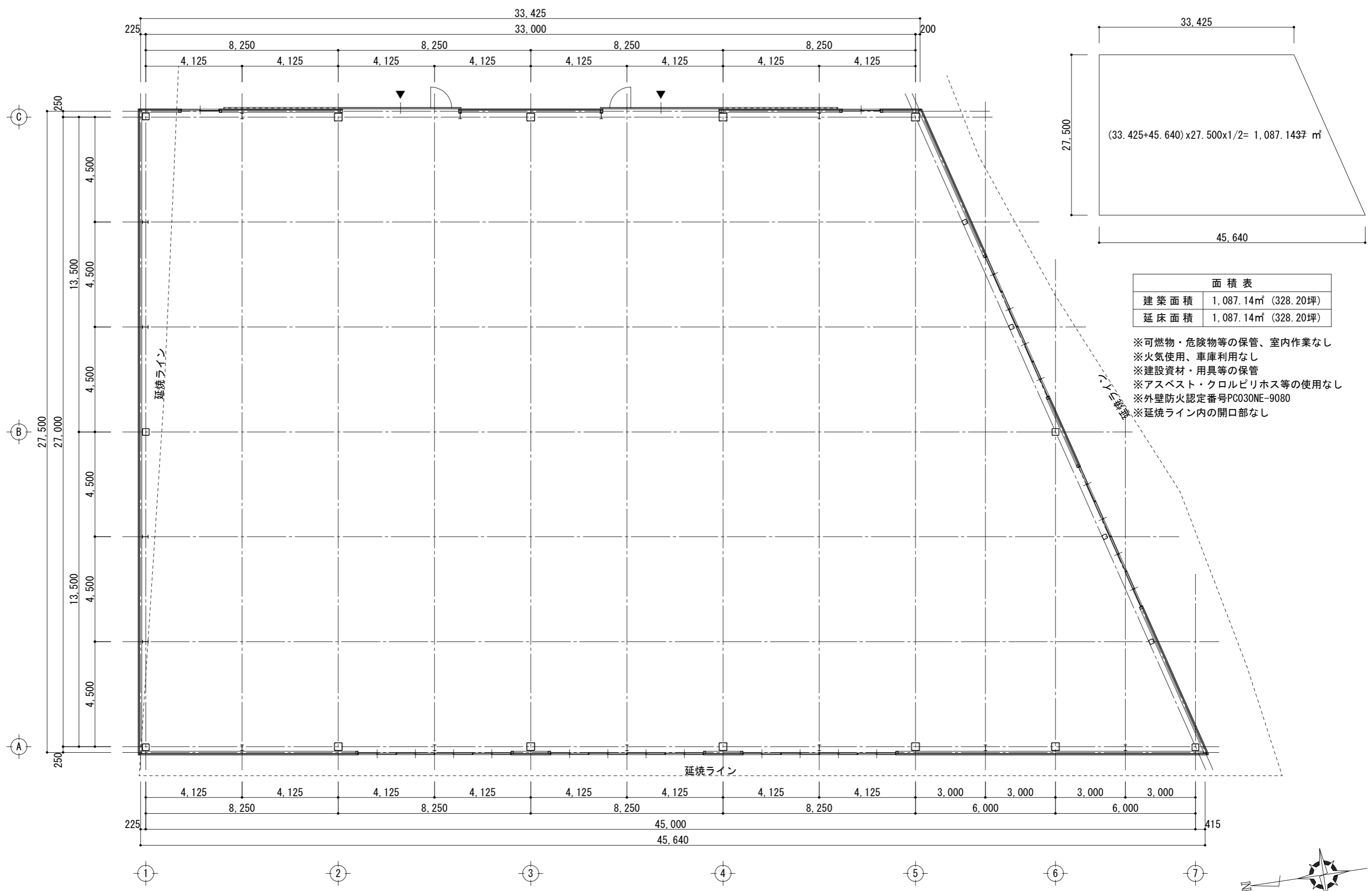
平面図 S=1:150
