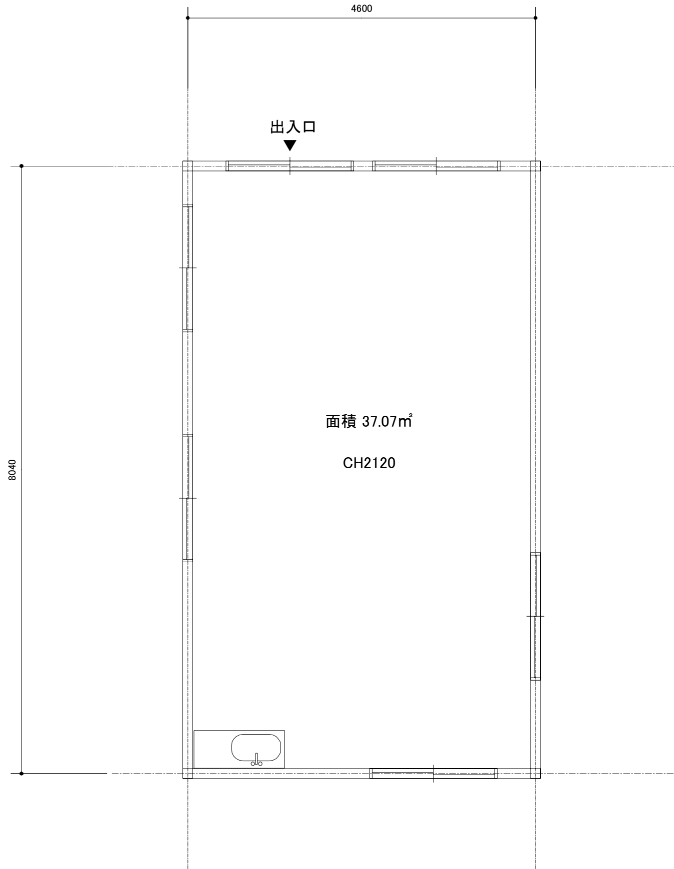
平面図 縮尺:1/50
